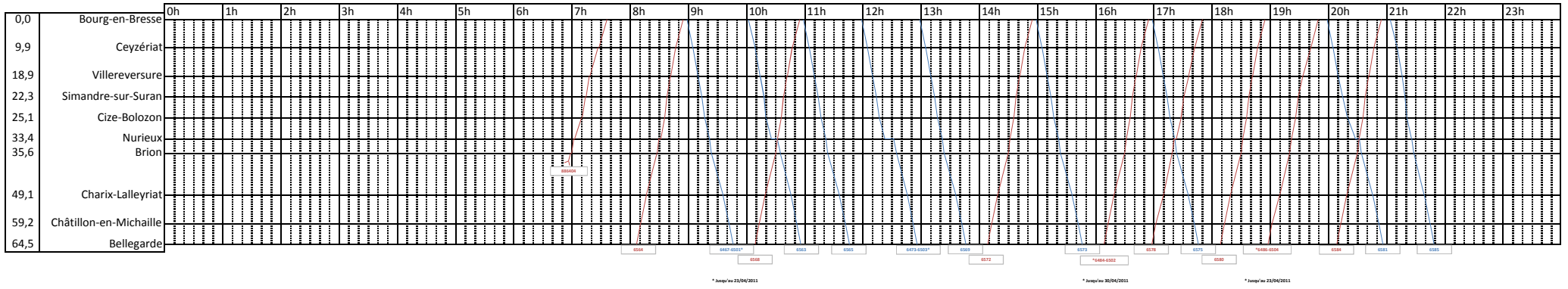
Graphique des circulations ligne Bourg-en-Bresse - Bellegarde - SA2011 (samedi)
