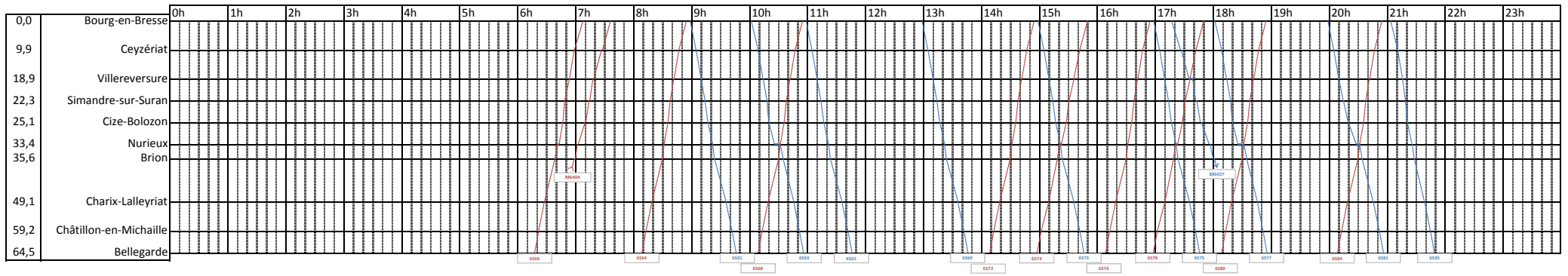
Graphique des circulations ligne Bourg-en-Bresse - Bellegarde - SA2011 (mardi)
